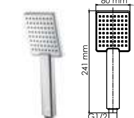
A141 Лейка 1-функциональная с системой защиты от известковых отложений
