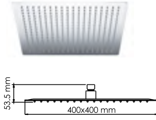
A119 Душевая насадка Нержавеющая сталь, 324 форсунок.
